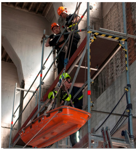
Personenrettung mit Schleifkorbtrage von einem Baugerüst
