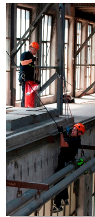
Ablassen des Retters zum Patienten
